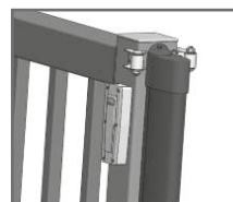
BARRE PALPEUSE EMBARQUÉE + KIT LIAISON MOBILE RADIO
