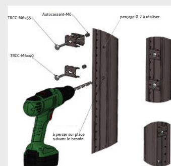
Montage simple
