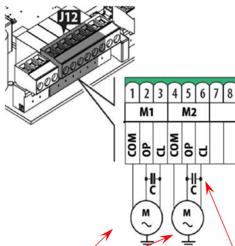
MOTEURS FAAC (Condensateurs à mettre dans le coffret)
