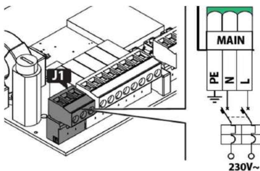
ALIMENTATION PRINCIPALE 220 V (P + N + Terre)
