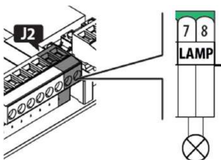
LAMPE CLIGNOTANTE (Attention au branchement dans la lampe)
